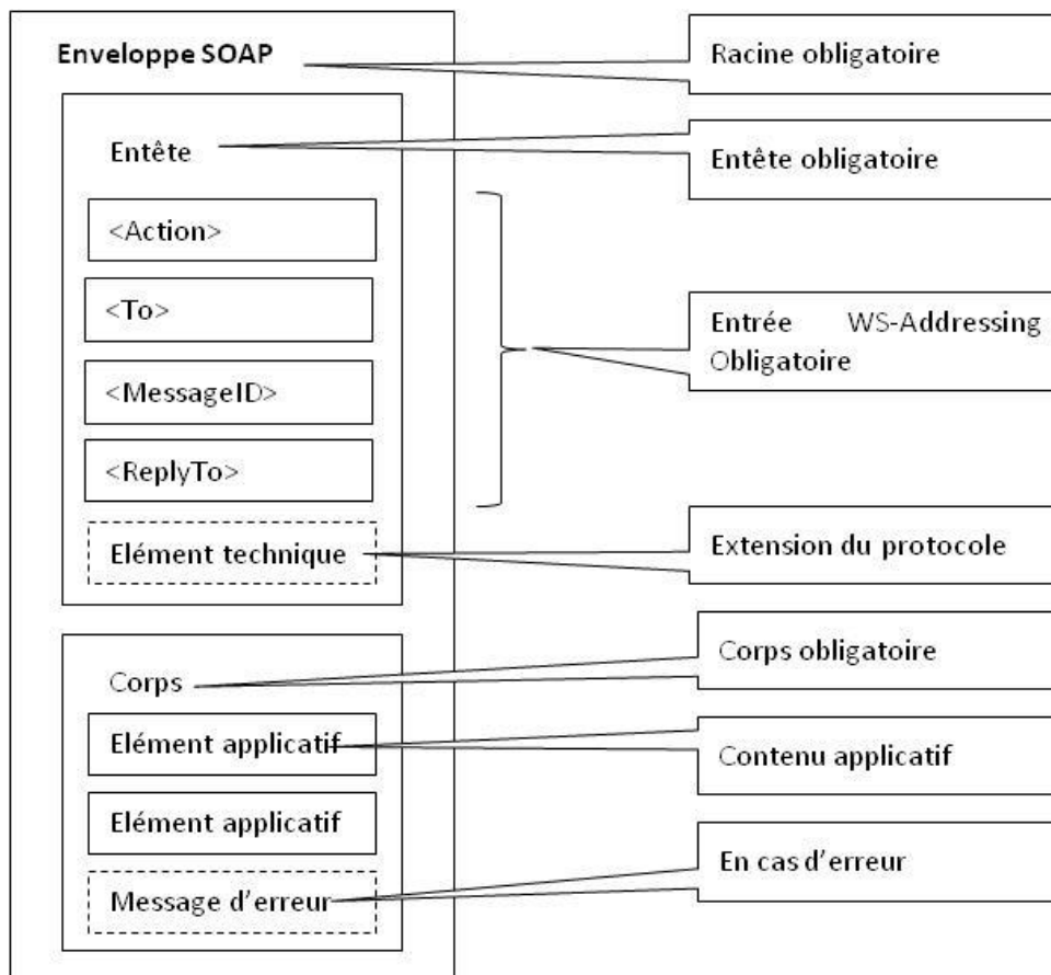
Figure 2 : Structure d'un message SOAP pour le cadre d'interopérabilité des SIS français
