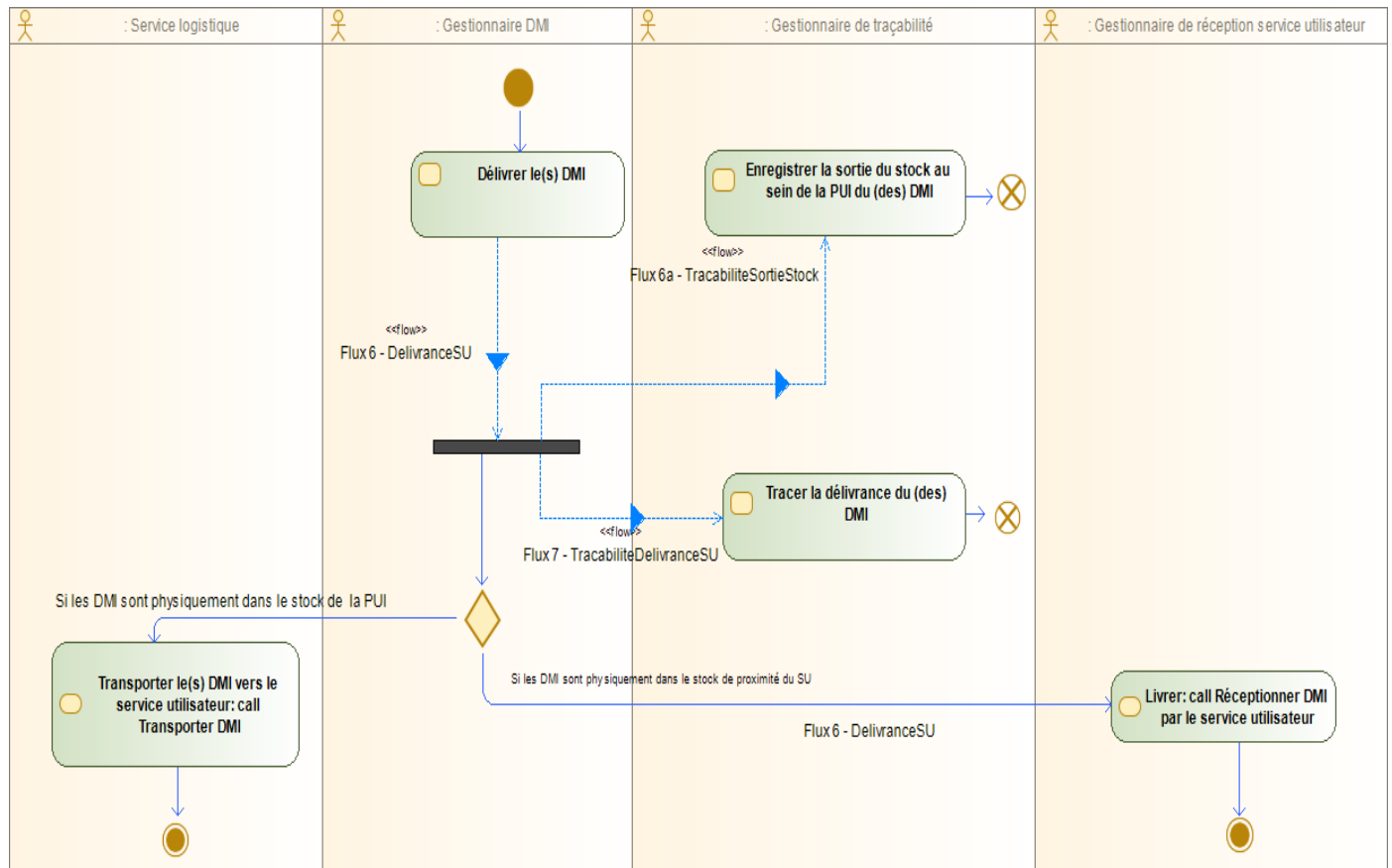
Figure 18 : Diagramme d'activité Délivrer DMI au Service Utilisateur
