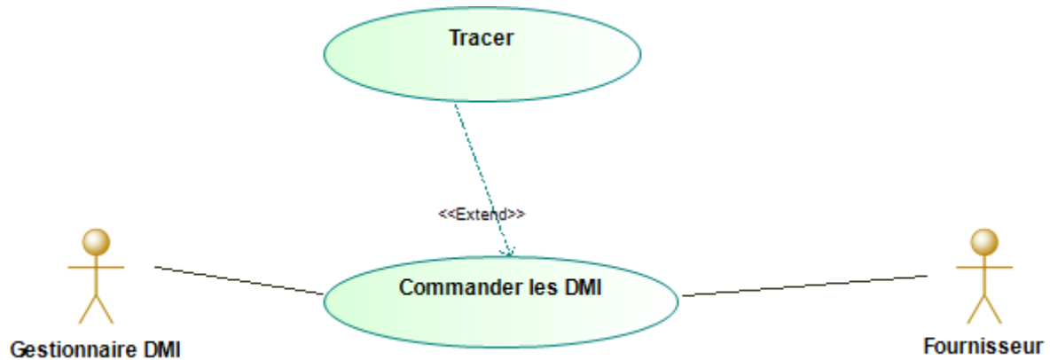
Figure 3 Cas d'utilisation "Commander les DMI"
