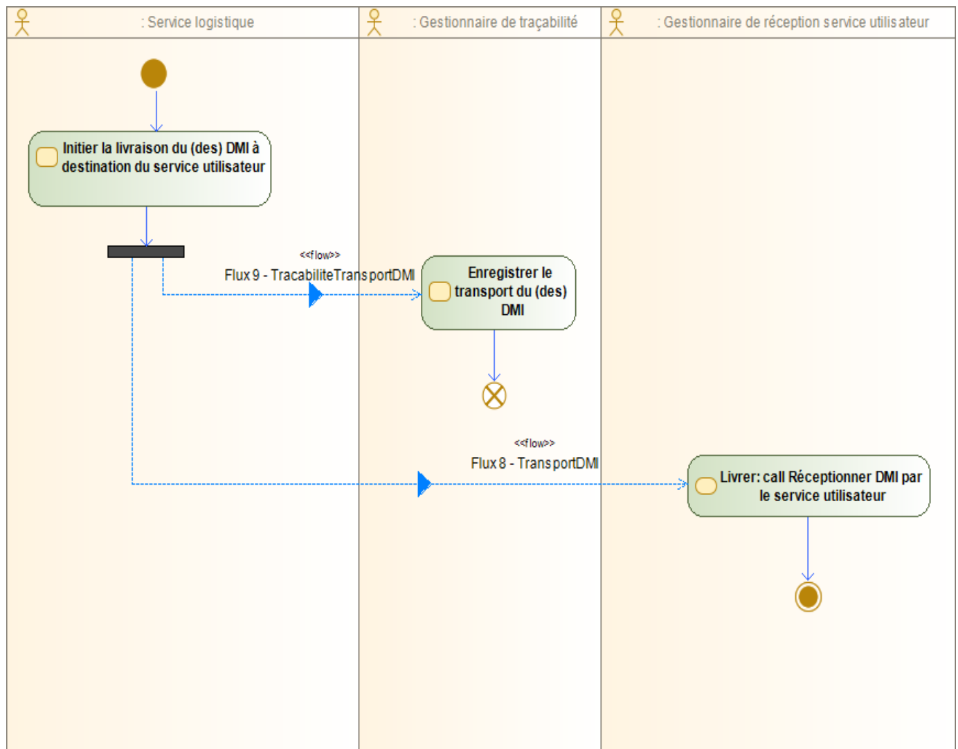
Figure 19 : Diagramme d'activité Transporter DMI
