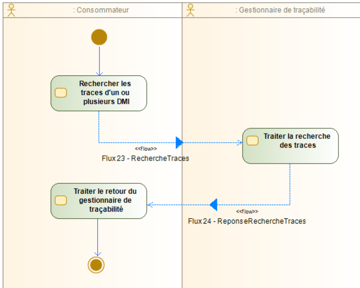
Figure 25 : Diagramme d'activité Rechercher des traces
