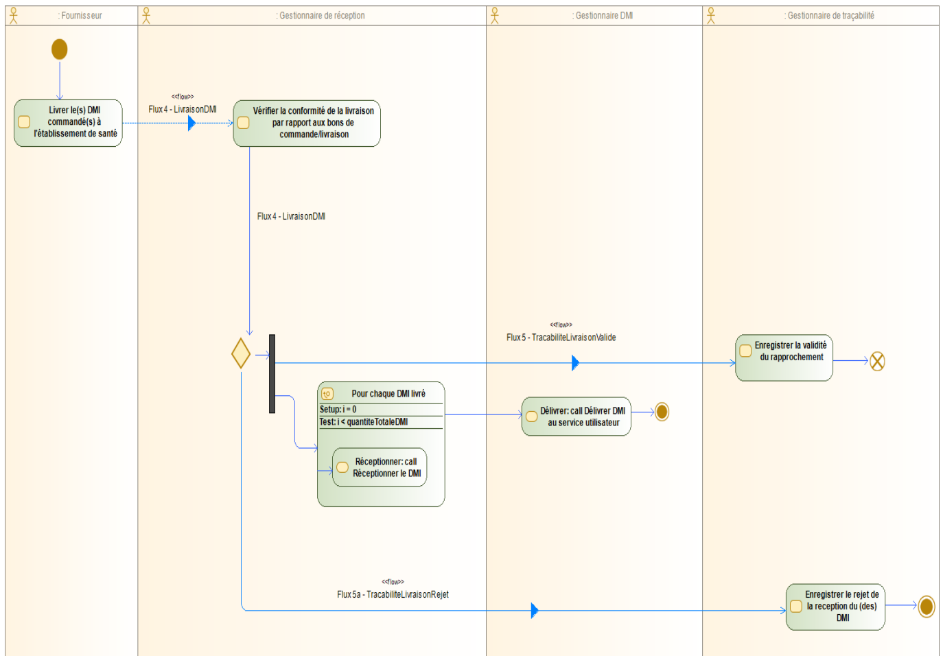
Figure 16 : Diagramme d'activité Réceptionner et contrôler DMI
