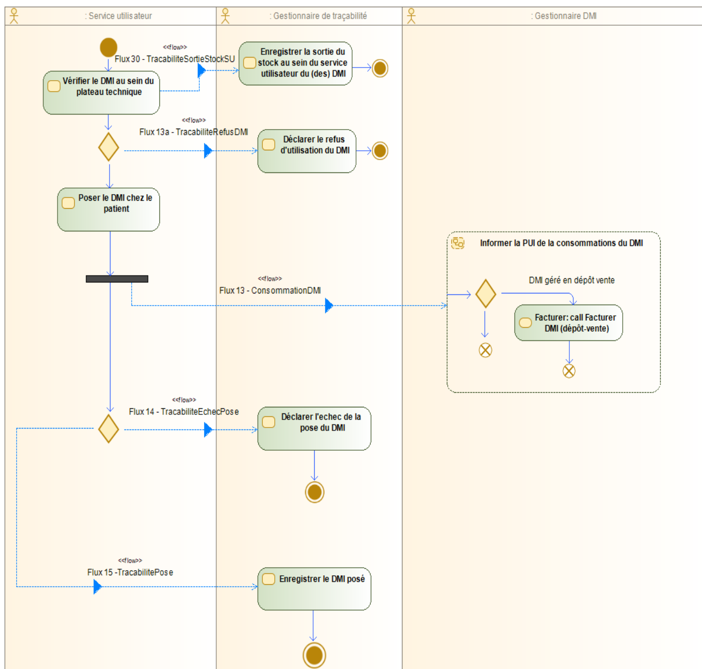
Figure 21 : Diagramme d'activité Poser DMI
