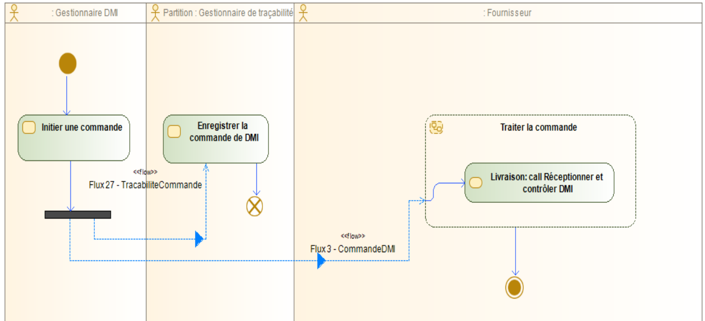
Figure 15 : Diagramme d'activité Commander les DMI
