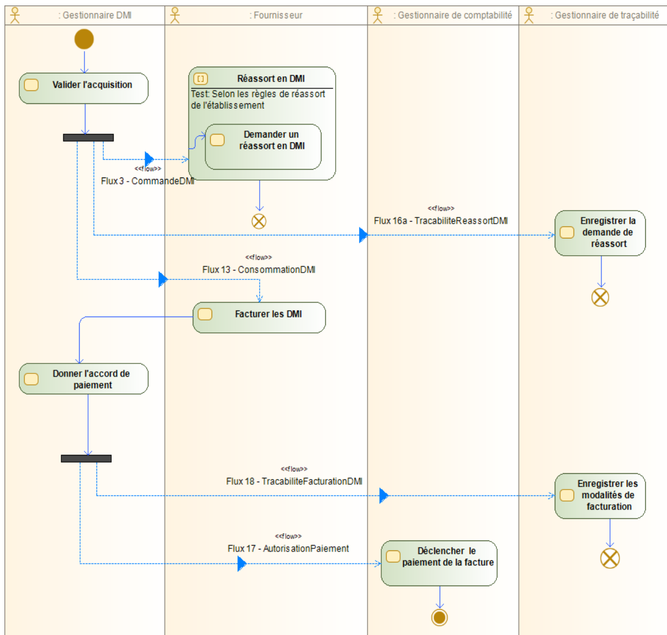
Figure 22 : Diagramme d'activité Facturer DMI (dépôt-vente)
