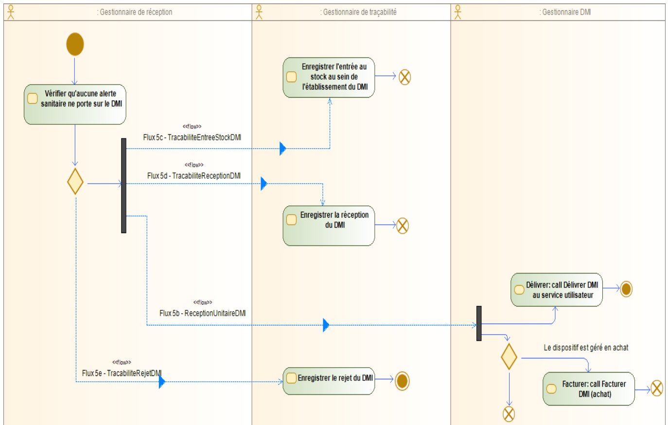
Figure 17 : Diagramme d'activité Réceptionner le DMI
