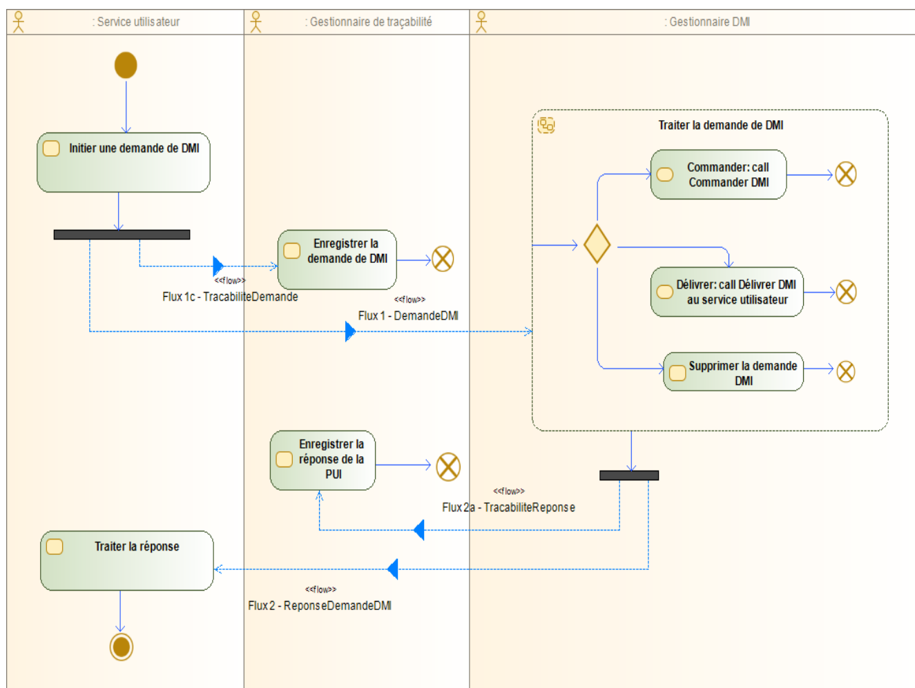
Figure 14 : Diagramme d'activité Demander DMI
