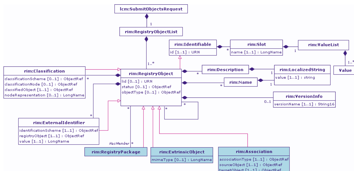
Les métadonnées XDS c'est-à-dire les attributs des classes XDS DocumentEntry, SubmissionSet, Folder ou Association, ont eux-aussi leur équivalent dans le modèle ebRIM.
