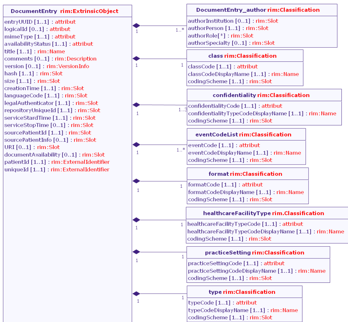
Figure 9: Equivalence attribut de DocumentEntry XDS – Objets ebRIM (en rouge)
